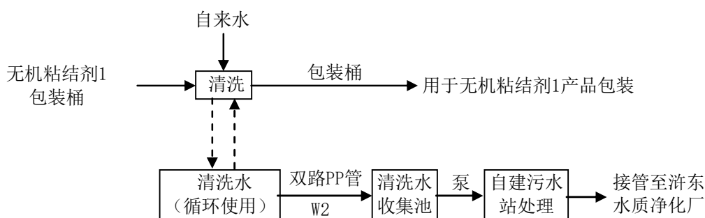
图 2-4 无机粘结剂（I）产品周转包装桶清洗工艺流程图
