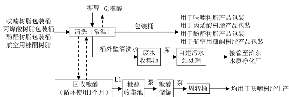
图 2-3 呋喃树脂/丙烯酸树脂/航空用糠酮树脂/酚醛树脂周转包装桶清洗工艺流程图
