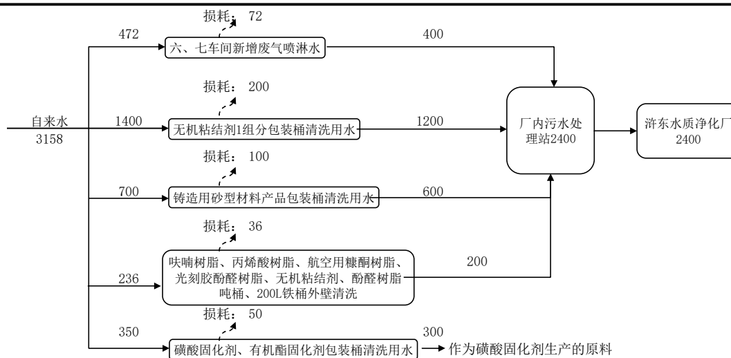
图 2-1 本次项目实际水平衡图 (t/a)
