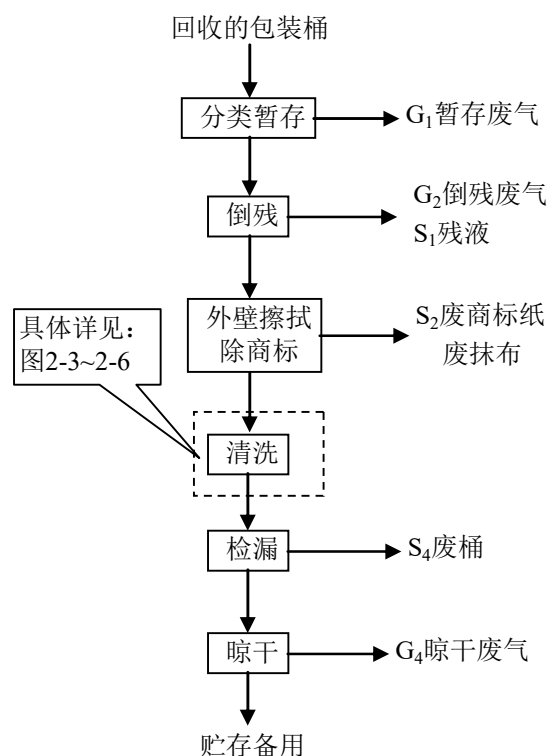
图 2-2 项目周转包装桶清洗总工艺流程图
