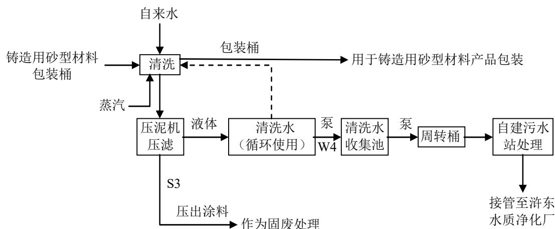
图 2-6 铸造用砂型材料产品周转包装桶清洗工艺流程图
