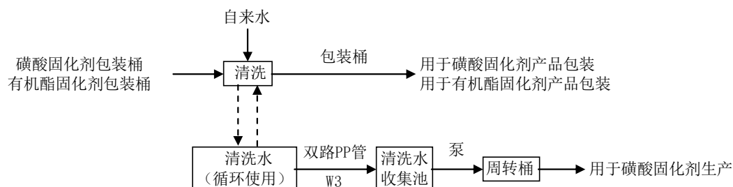
图 2-5 磺酸固化剂/有机质固化剂产品周转包装桶清洗工艺流程图
